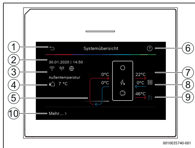
Bild 6 Anlagenübersicht
