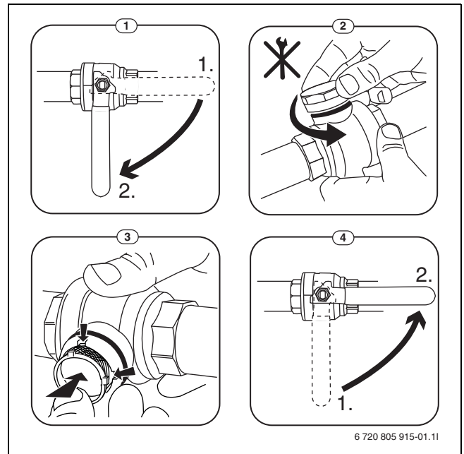
Bild 7 Siebreinigung
