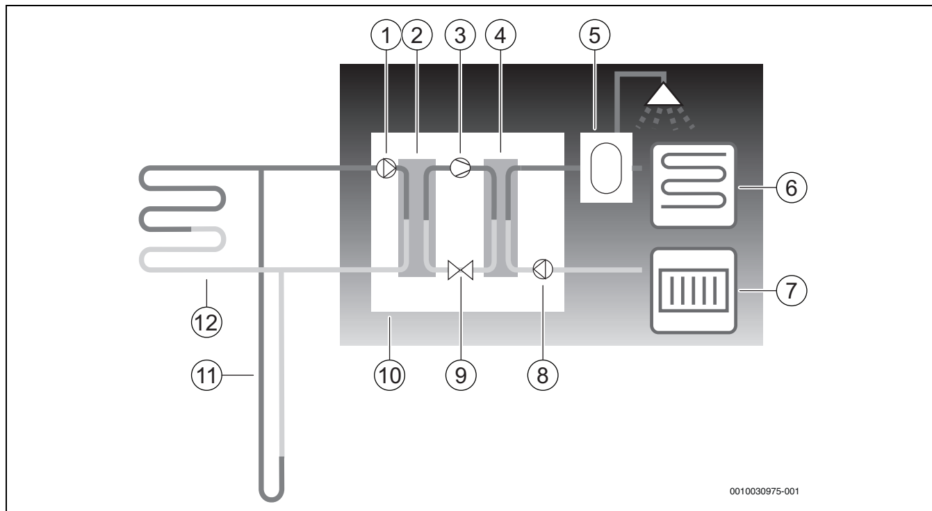
Bild 1 Funktionsbeschreibung
