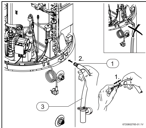
Bild 12 Kondensatauffang
