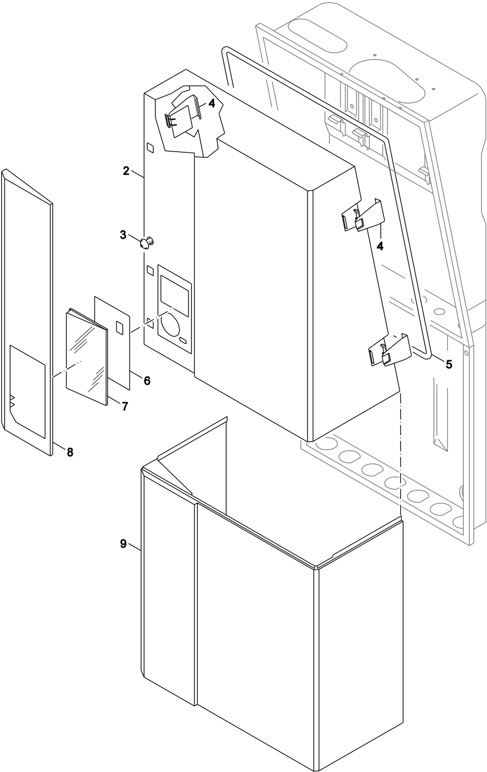
6720906451.ab.RS-Verkleidung GB112 24/24T 25/
