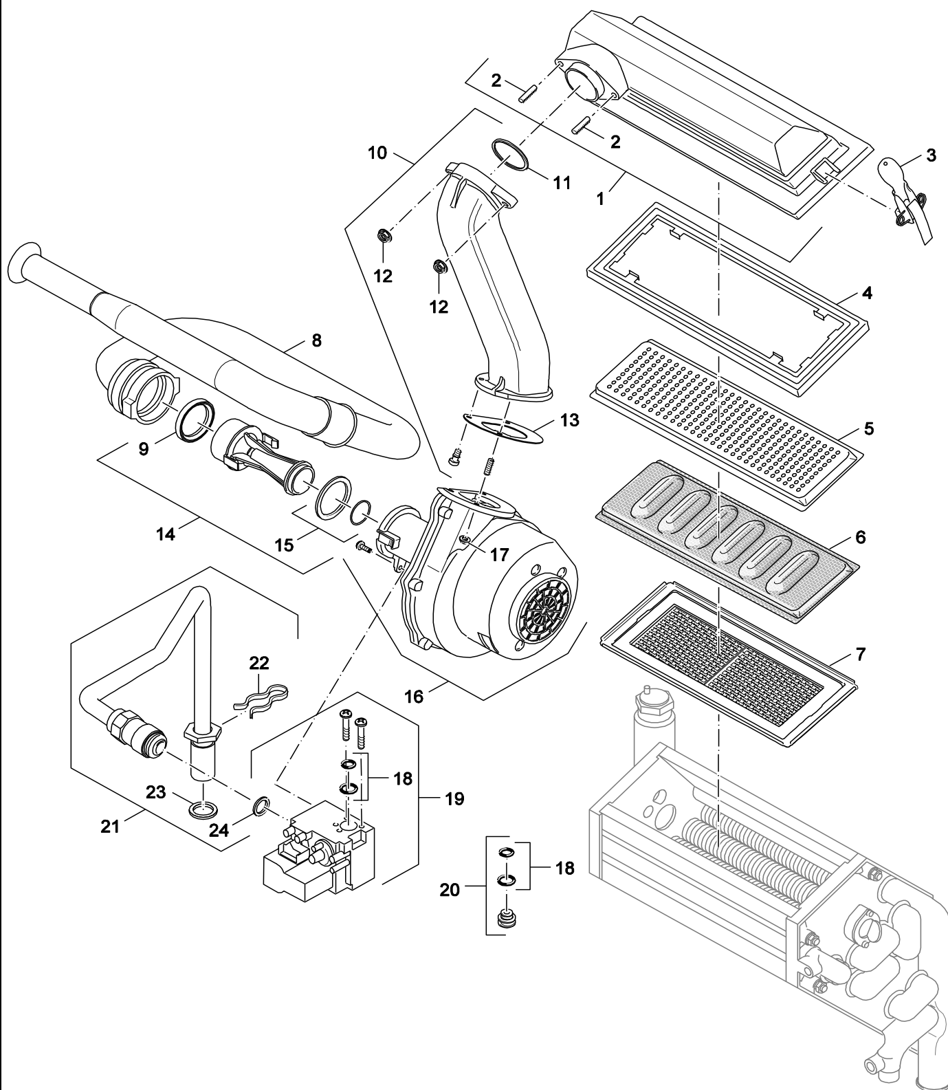
6720905714.aa.RS-Brennereinheit/Gebläse/Gasarmatur GB142 15/24/30
