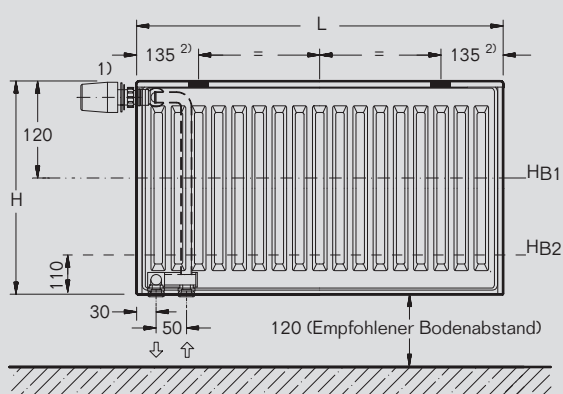
Rückansicht Typ 20/21/22/30/33
