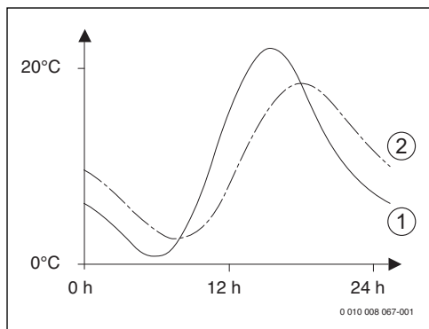
Bild 11 Beispiel für die gedämpfte Außentemperatur
