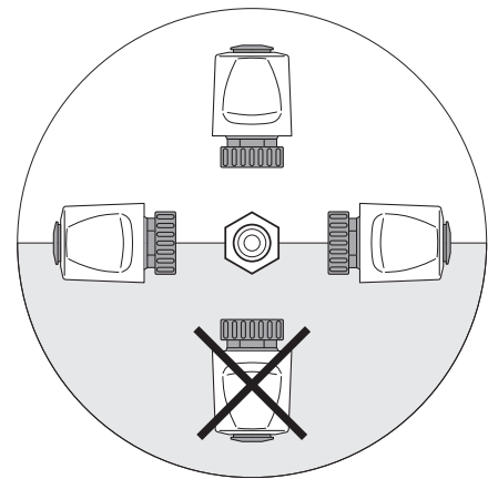
Einbaulagen
