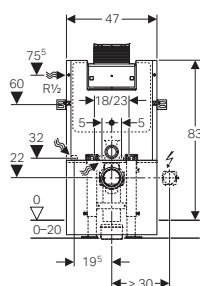
Geberit Sanbloc → Art.Nr. 440.000.00.1 BH 83 cm
