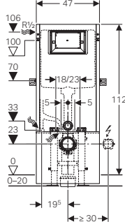
Geberit Sanbloc → Art.Nr. 440.010.00.1 BH 112 cm
