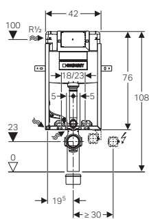
Geberit Kombifix → Art.Nr. 110.020.00.1 BH 108 cm
