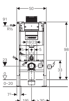
Geberit Duofix → Art.Nr. 111.030.00.1 BH 98 cm
