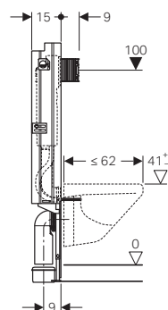
Geberit Sanbloc → Art.Nr. 440.010.00.1 BH 112 cm
