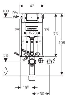
Geberit Kombifix → Art.Nr. 110.020.00.1 BH 108 cm
