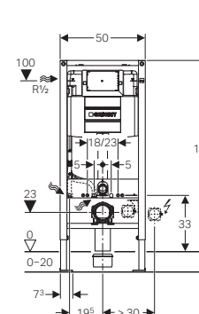
Geberit Duofix → Art.Nr. 111.060.00.1 BH 112 cm
