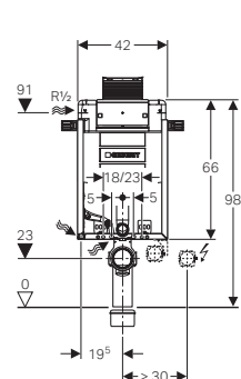
Geberit Kombifix → Art.Nr. 110.010.00.1 BH 98 cm
