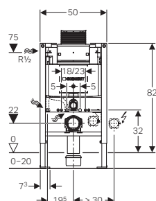
Geberit Duofix → Art.Nr. 111.003.00.1 BH 82 cm
