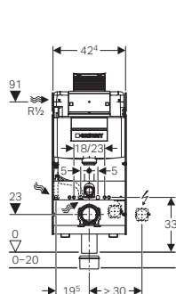
Geberit GIS → Art.Nr. 461.151.00.1 BH 100 cm
