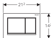
Geberit Omega30 → Art.Nr. 115.080.xx.1
