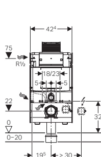
Geberit GIS → Art.Nr. 461.141.00.1 BH 87 cm
