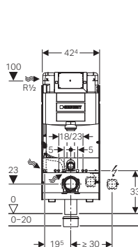
Geberit GIS → Art.Nr. 461.160.00.1 BH 114 cm
