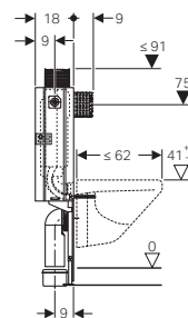
Geberit Sanbloc → Art.Nr. 440.000.00.1 BH 83 cm
