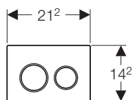
Geberit Omega20 → Art.Nr. 115.085.xx.1
