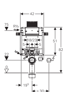
Geberit Kombifix → Art.Nr. 110.000.00.1 BH 82 cm
