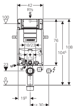
Geberit Kombifix für Geruchsabsaugung Abluft → Art.Nr. 110.367.00.5
