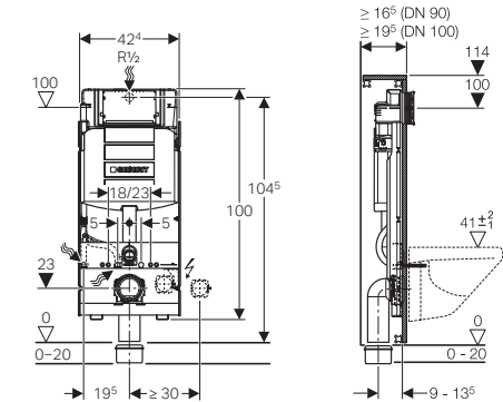
Geberit GIS → Art.Nr. 461.311.00.5 461.303.00.5 GIS WC-Eckmodul
