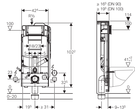
Geberit GIS für Geruchsabsaugung Umluft → Art.Nr. 461.370.00.5
