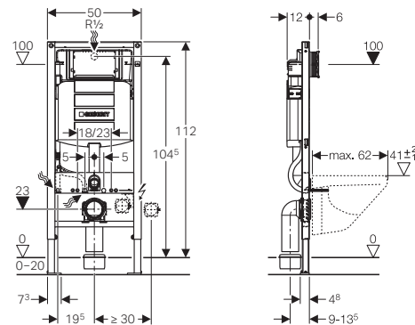
Geberit DuoFix → Art.Nr. 111.300.00.5 111.350.00.5 111.385.00.5 111.396.00.5 111.390.00.5 111.375.00.5 111.914.00.5 barrierefrei, höhenverstellbar 5 cm, Rohbau Breite variabel, 80–120 cm Nachträglich höhenverstellbar um 8 cm Eckelement Für Stütz- und Haltegriffe Kinder-WC
