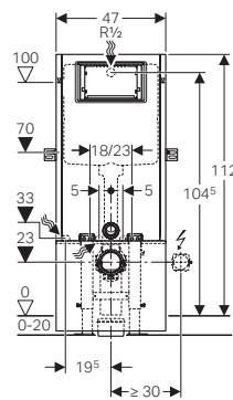
Geberit Sanbloc
