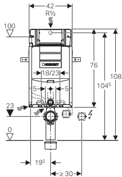
Geberit Kombifix Plus → Art.Nr. 110.300.00.5
