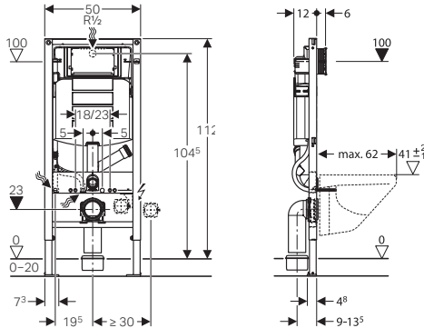
Geberit DuoFix für Geruchsabsaugung Abluft → Art.Nr. 111.364.00.5
