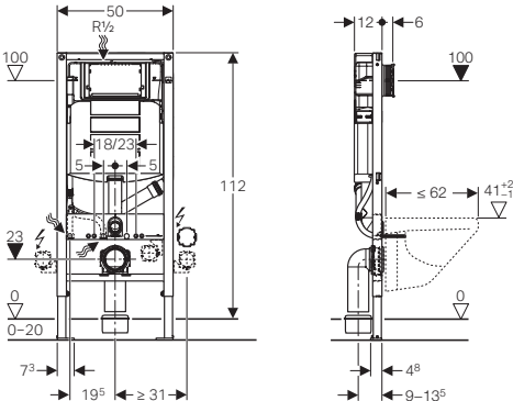
Geberit DuoFix für Geruchsabsaugung Umluft → Art.Nr. 111.370.00.5
