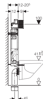
Geberit Kombifix für Geruchsabsaugung Abluft → Art.Nr. 110.367.00.5
