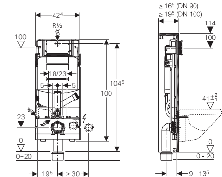
Geberit GIS für Geruchsabsaugung Abluft → Art.Nr. 461.315.00.5
