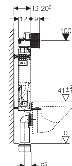
Geberit Kombifix für Geruchsabsaugung Abluft → Art.Nr. 110.367.00.5
