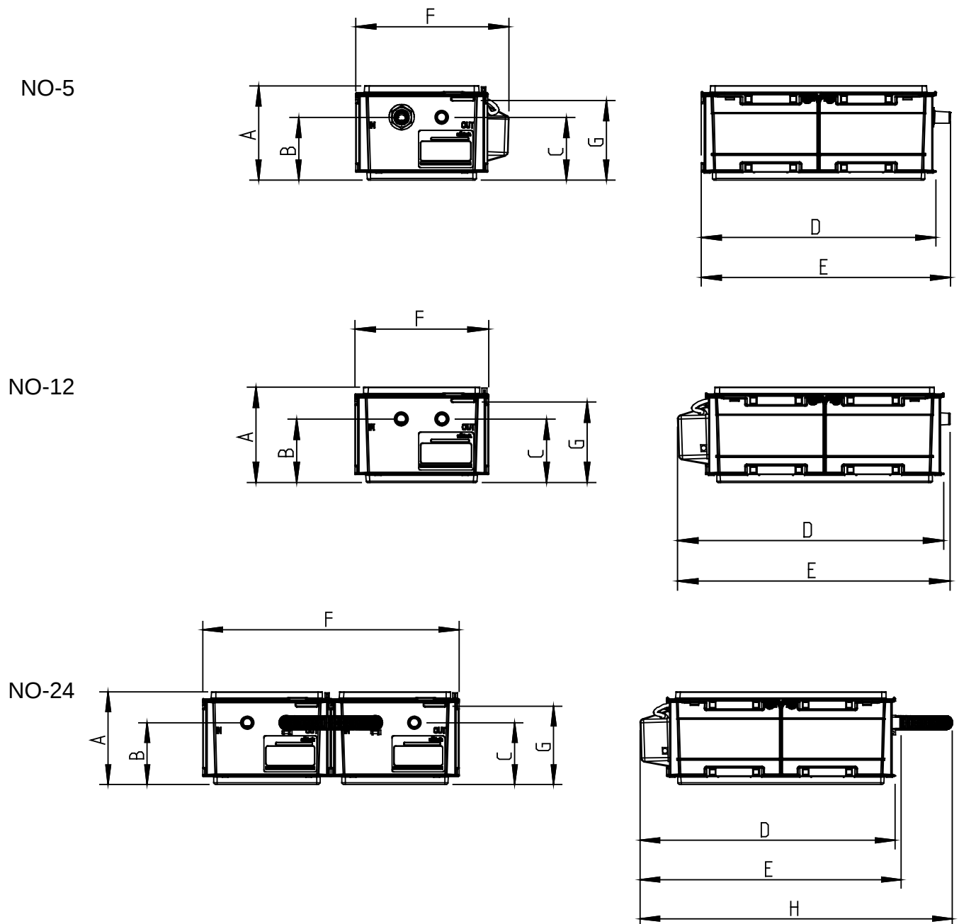
Abb. C-4: Maßzeichnung
