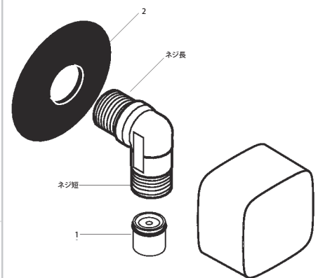
製品分解図
