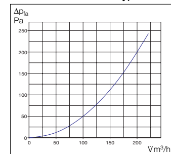
Druckverlust-Volumenstrom Type VFE 70 Type VFE 90
