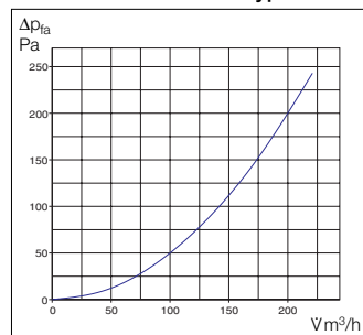
Druckverlust-Volumenstrom Type VFE 70 Type VFE 90
