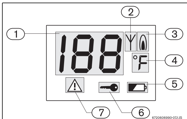
Fig. 25 LCD multifonctionnel
