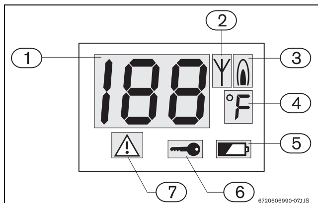
Fig. 17 Pantalla LCD multifuncional
