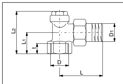
Modèle équerre avec filetage femelle
