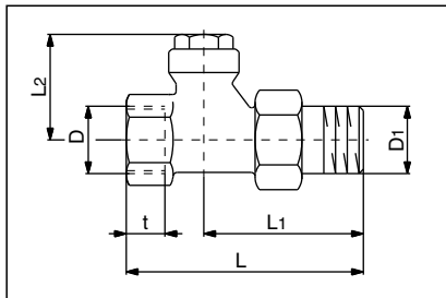
Durchgangsform mit Innengewinde
