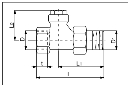
Modèle droit avec filetage femelle
