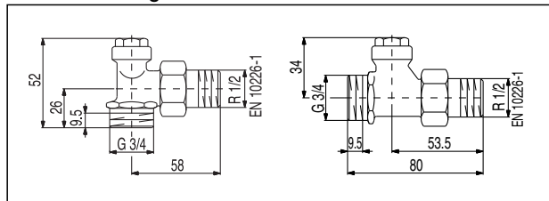
«Combi 4» filetage mâle des deux côtés
