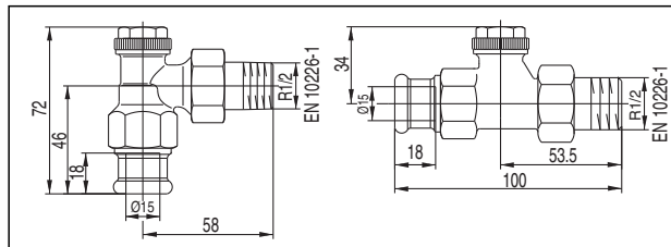
«Combi 3» avec raccordement à sertir
