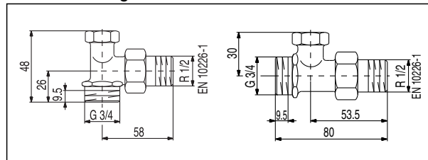
«Combi 2» filetage mâle des deux côtés
