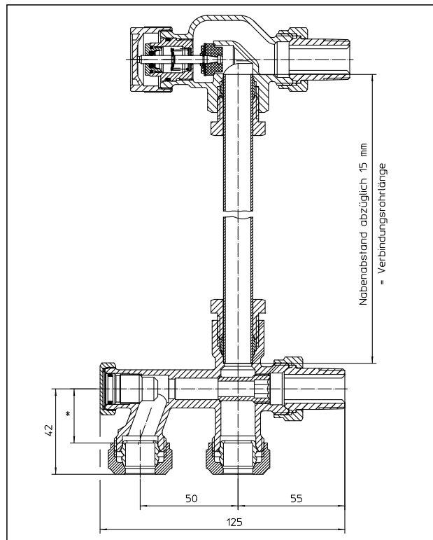
„Bypass-Combi Duo“ mit Vorlauf-Axialventil
