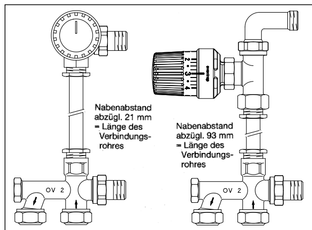
„Bypass-Combi Duo“ mit Winkeleckventil
