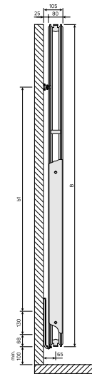
Vertical 2024 Seitenansicht Typ 20
