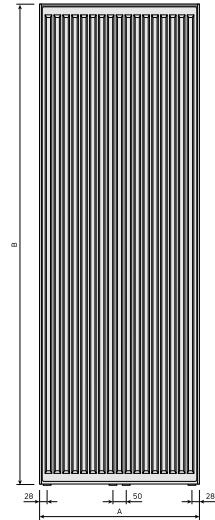
Vertical 2024 Frontansicht Typen 20, 21 und 22
