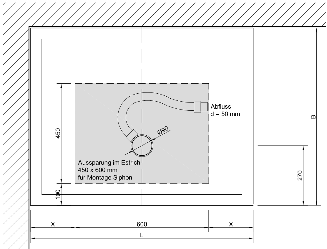
Grundriss | 1:10
