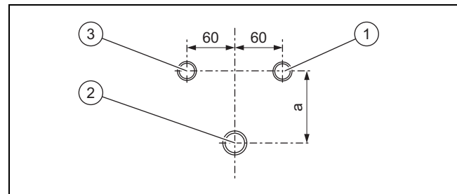
Unterputzinstallation
