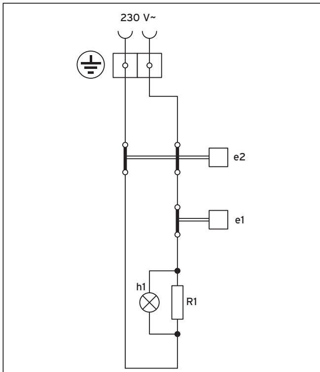
Abb. 5.1 Schaltschema
