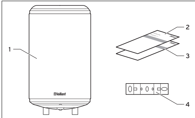
Abb. 4.1 Lieferumfang
