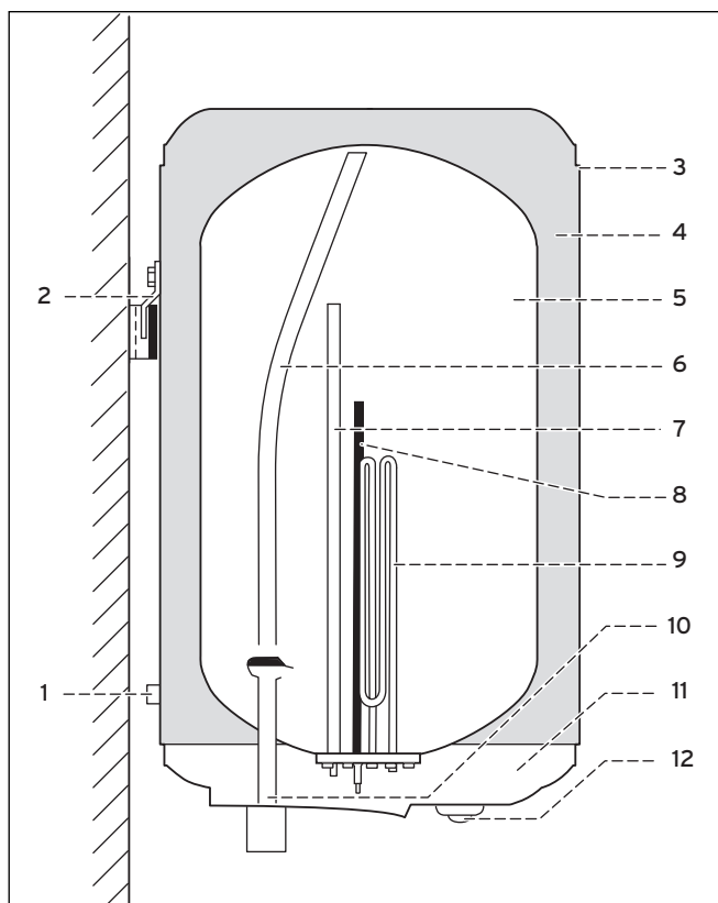
Abb 3.1 Übersicht
