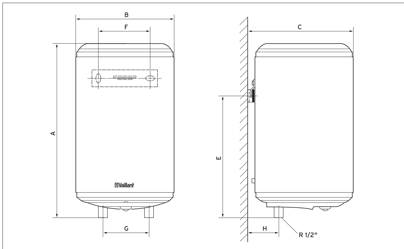
Abb. 4.2 Geräteabmessungen
