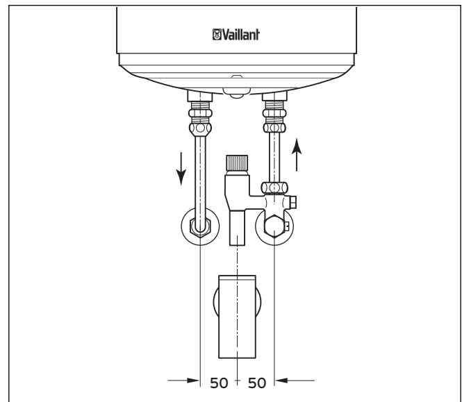
Abb. 4.3 Vorderansicht bei geschlossenem System (Maße in mm)
