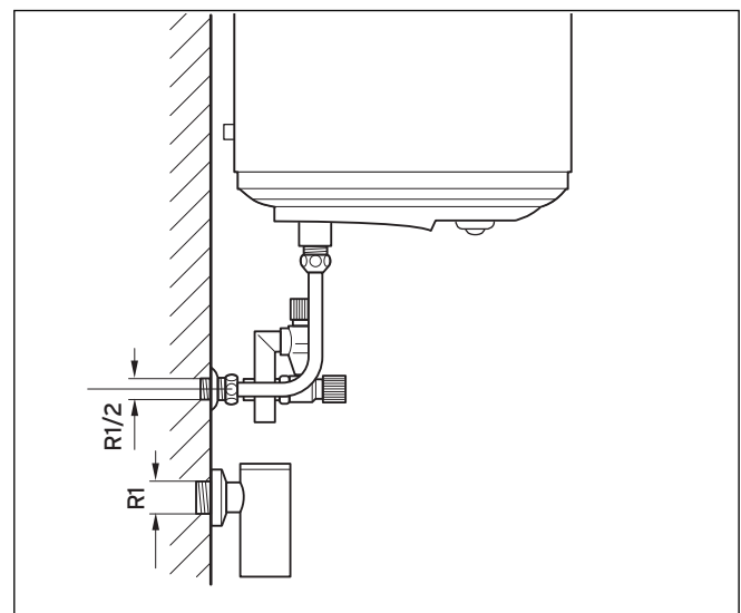
Abb. 4.4 Seitenansicht bei geschlossenem System
