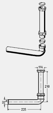
Ablaufbogen 90° - Kunststoff Ausstattung Ablaufrohr Modell 5632.2
