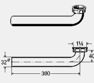
Ablaufbogen 90° - Kunststoff Modell 5621.25
