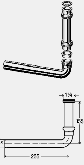
Ablaufbogen 90° - Messing verchromt Modell 5621.1-880
