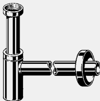
Eleganta 1-Flaschengeruchverschluss - Messing verchromt Ausstattung Verstellrohr 200 mm, Ablaufrohr 310 mm, Rosette Ø32xØ80xH15 mm Modell 5788
