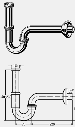
Röhrengeruchverschluss Plus-Siphon - Messing Ausstattung Verstellrohr 120 mm, Ablaufbogen 220 mm güteüberwacht nach DIN EN 274 Modell 5611.5
