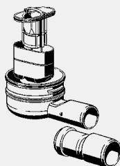
Advantix-Duschrinnen-Geruchverschluss - für Einbauhöhe ab 95 mm - nachträglich als Sanierungsmodell kürzbar
