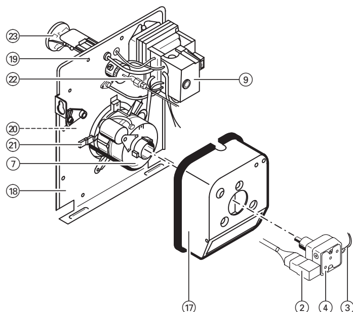
Abb. 18 Gebläsemotor
