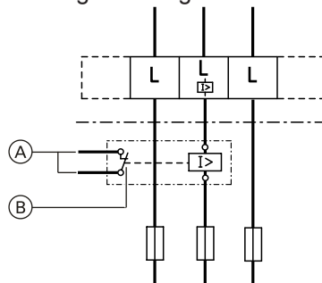
Ⓐ Steuerleitung zum Schaltschütz des 2. Gerätes (z. B. Elektro-Speicherheizgerät). Ⓑ Steuerkontakt öffnet beim Einschalten des Durchlauferhitzers.
